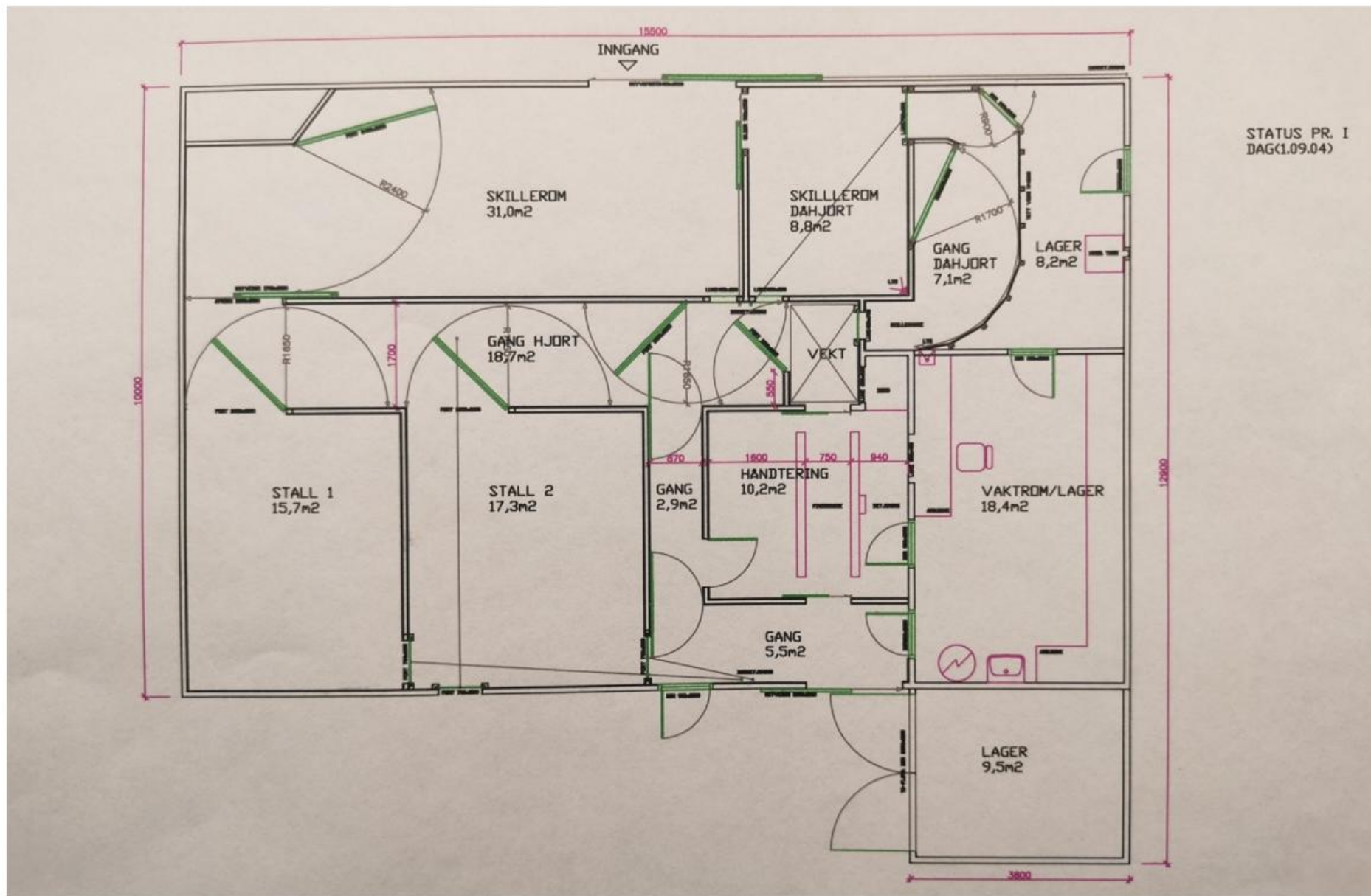
Figur 1. Planteikning av handteringsanlegget ved Norsk Hjortesenter. Utandørs drivgangar omtalt i teksten kjem inn frå hjørnet need til høgre, går langs veggjen til høgre og oppe i figuren.
